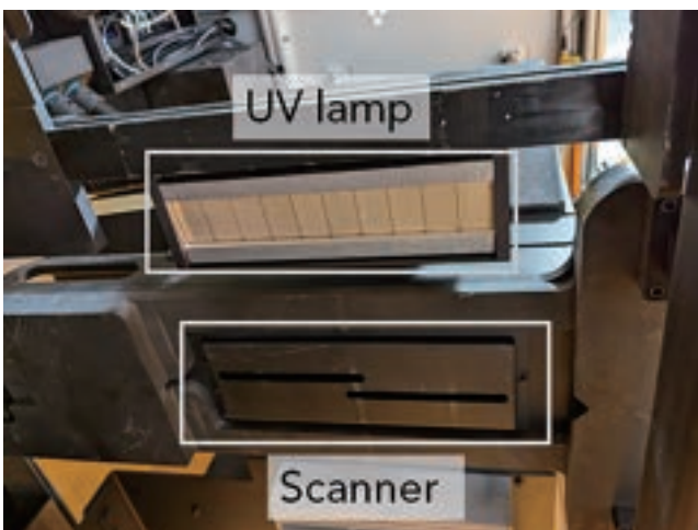
図3 VCJスキャナーシステムを備えたインクビット社の3Dプリンターモジュール
