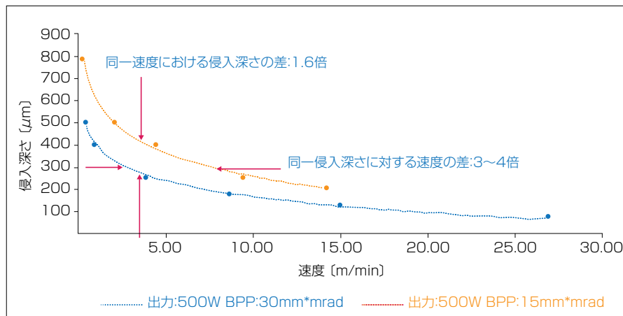
図4 純銅の溶接速度と侵入深さに対するBPPの影響
