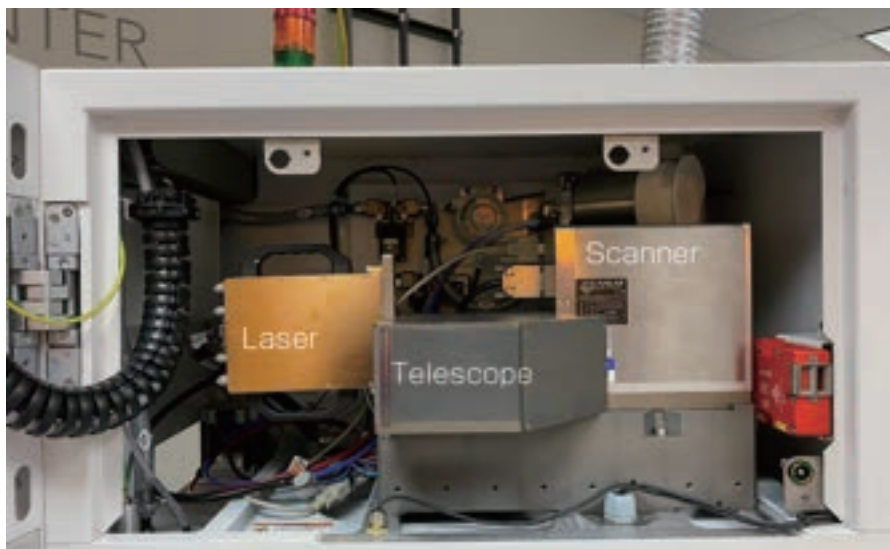
図5 商用粉末床3Dプリンター内部に統合されたレーザモジュール、ビームエキスパンダー、スキャナ
