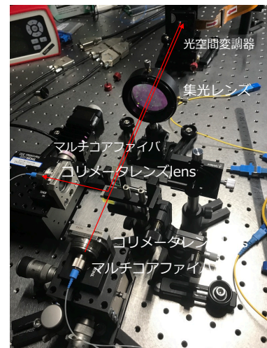
図3 コア選択スイッチの原理確認実験の様子
