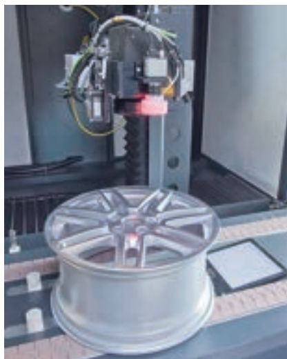
図2 光学式部品認識、自動搬送、レーザー加工、品質検査などの、自動車ホイール加工用統合レーザー装置。
