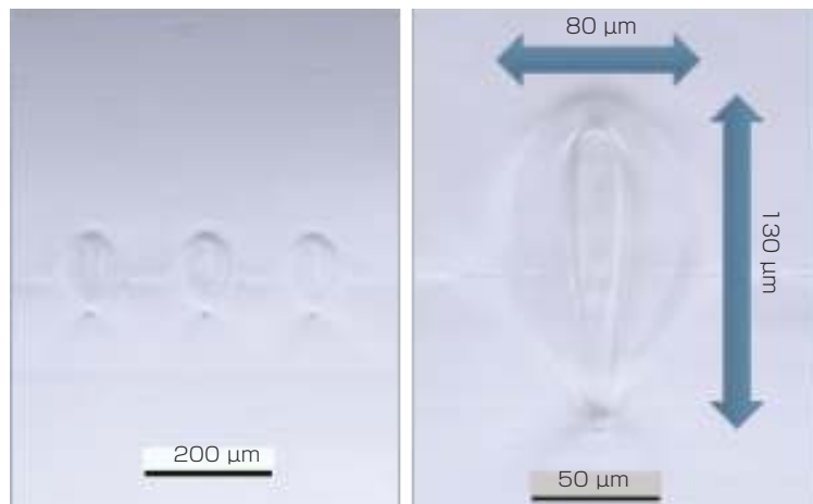
図3 左は、約 200\mu\text{m} の中心間隔で並ぶガラス微細溶接ラインで、右は、さらなる細部を示したその拡大写真。
