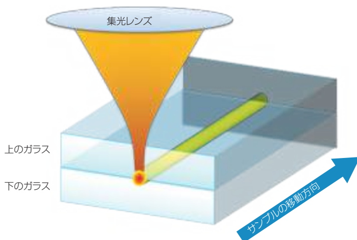
図1 2枚のガラス板に対する透過型レーザ微細溶接の概念図。
